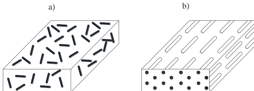
Rys. 1. Schemat kompozytu o budowie a) stochastycznej, b) deterministycznej
